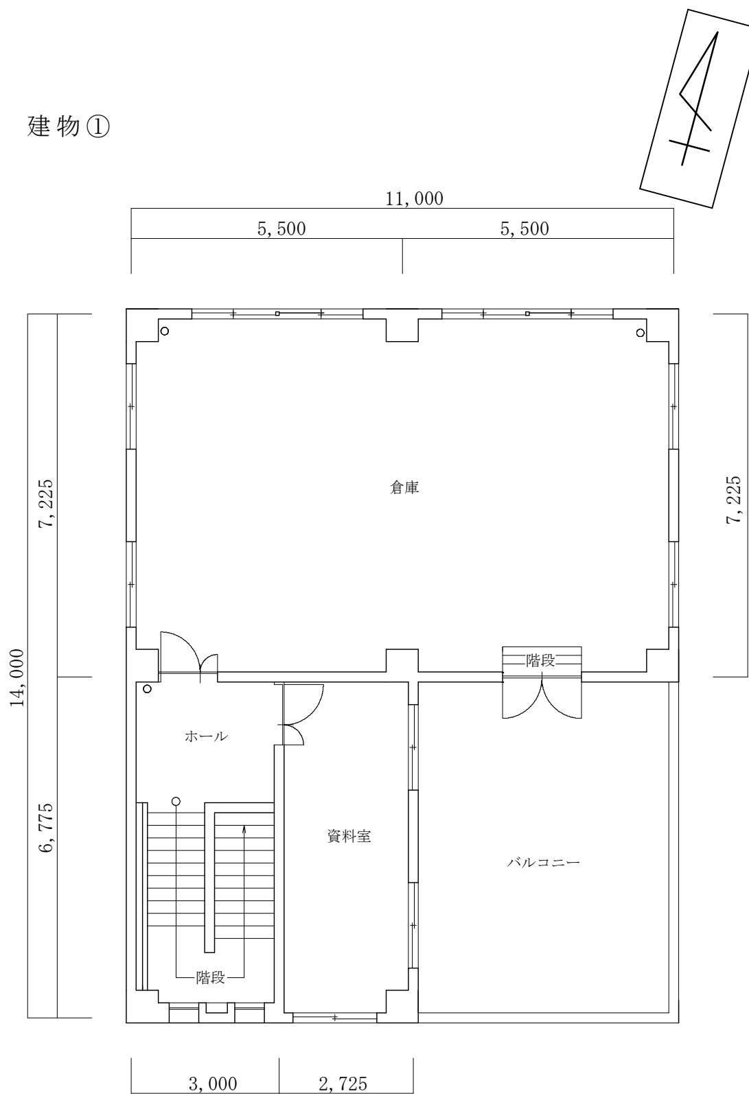
2 階 平 面 図
