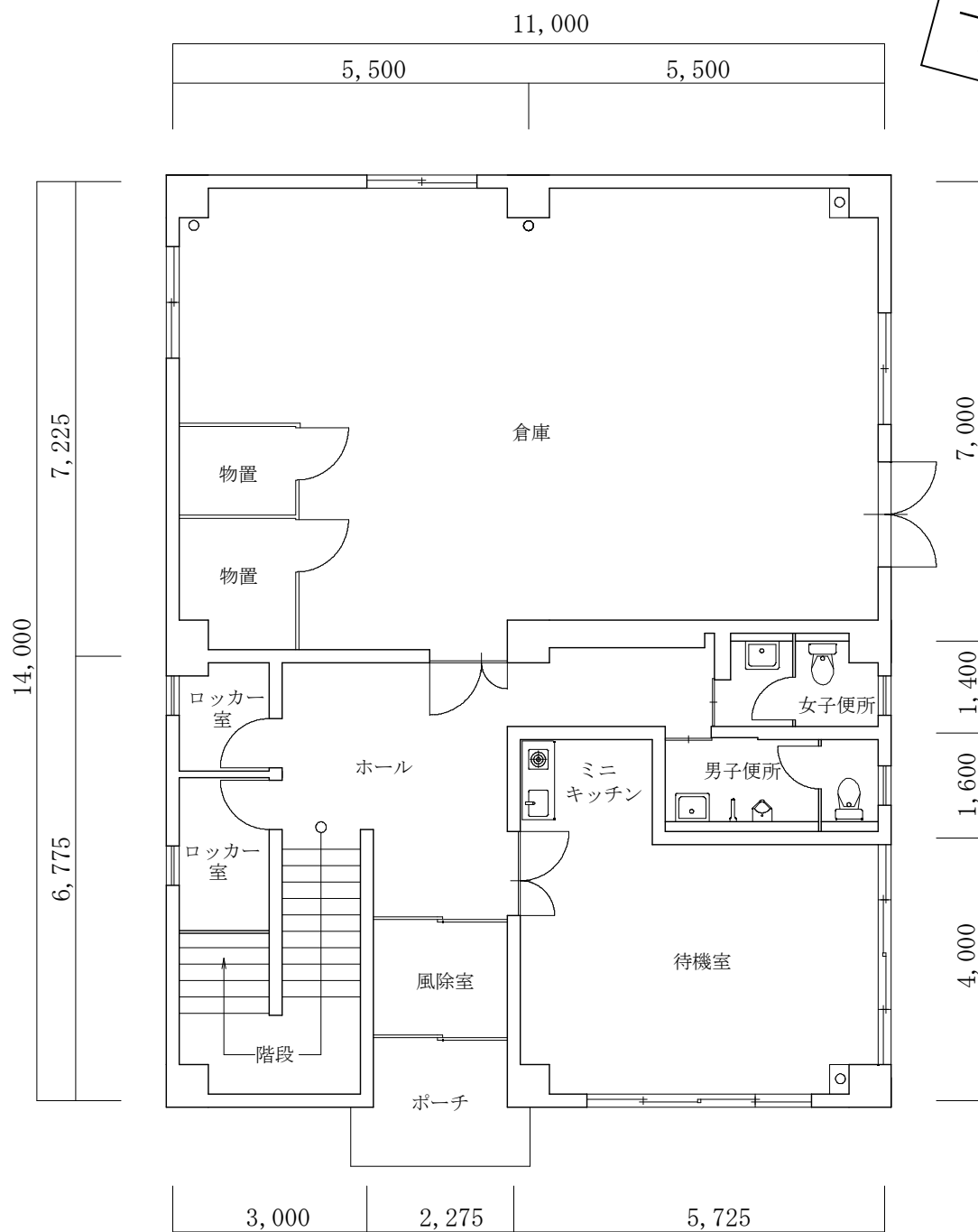
1 階 平 面 図
