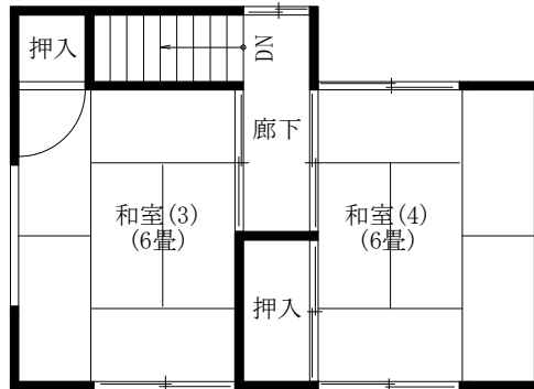
2 階平面図
