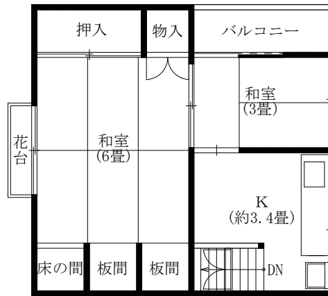
2階平面図
