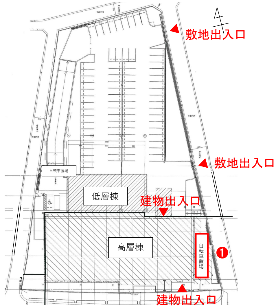
建物配置図
