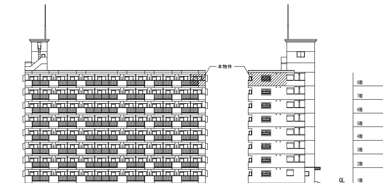
南東側立面図
